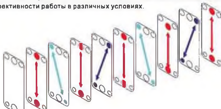
Двухходовая схема
