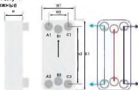
К215: Двухходовая схема - 6 подсоединений
